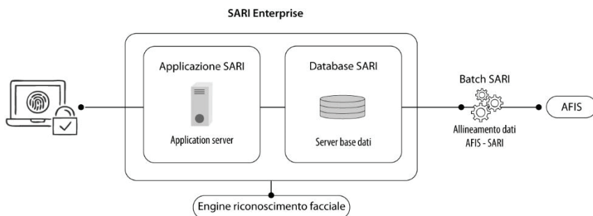
Figura 1: architettura logica di SARI Enterprise
